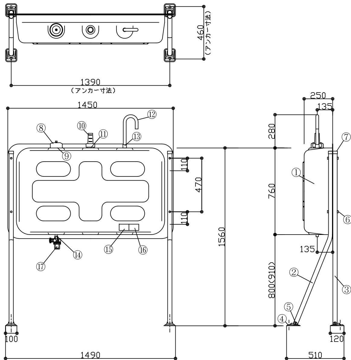
〈 〉内寸法は取付位置を上げた場合
